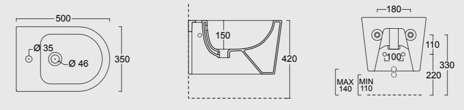
Bidet sospeso Form Form bidet wall hung
