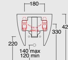
Cod. 45010101 Bidet sospeso Wunder Wunder bidet wall hung
